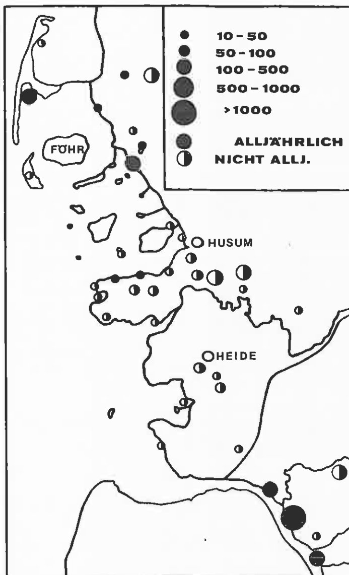
Die maximalen Bestände des Zwergschwans an der Westküste Schleswig-Holsteins 1965 - 1977.
